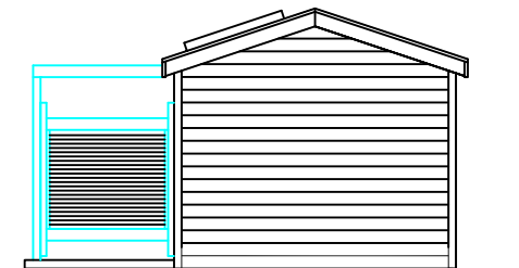
RIGHT ELEV.
