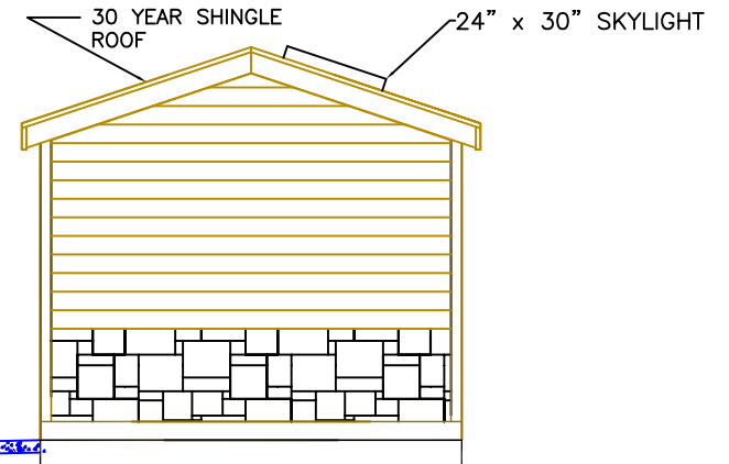
RIGHT ELEV.
