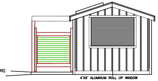
RIGHT ELEV.
