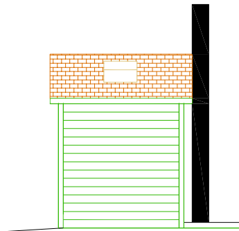
RIGHT ELEV.
