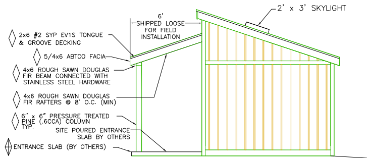
RIGHT ELEV.
