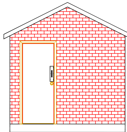
RIGHT ELEVATION
