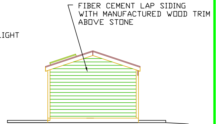
RIGHT ELEVATION
