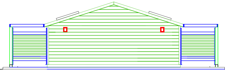
RIGHT END ELEVATION
