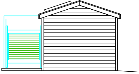
RIGHT ELEV.
