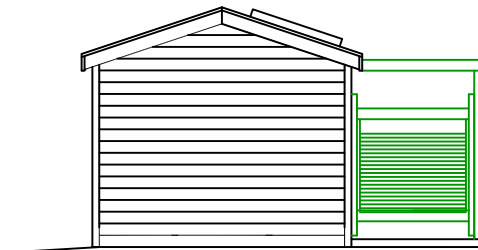
END ELEVATION
