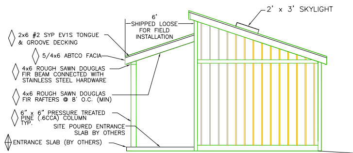
RIGHT ELEV.
