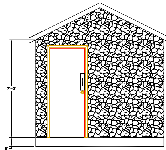
RIGHT ELEVATION
