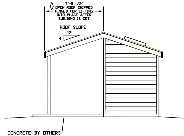
RIGHT ELEV.
